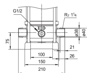
Conexión roscada (/G)
