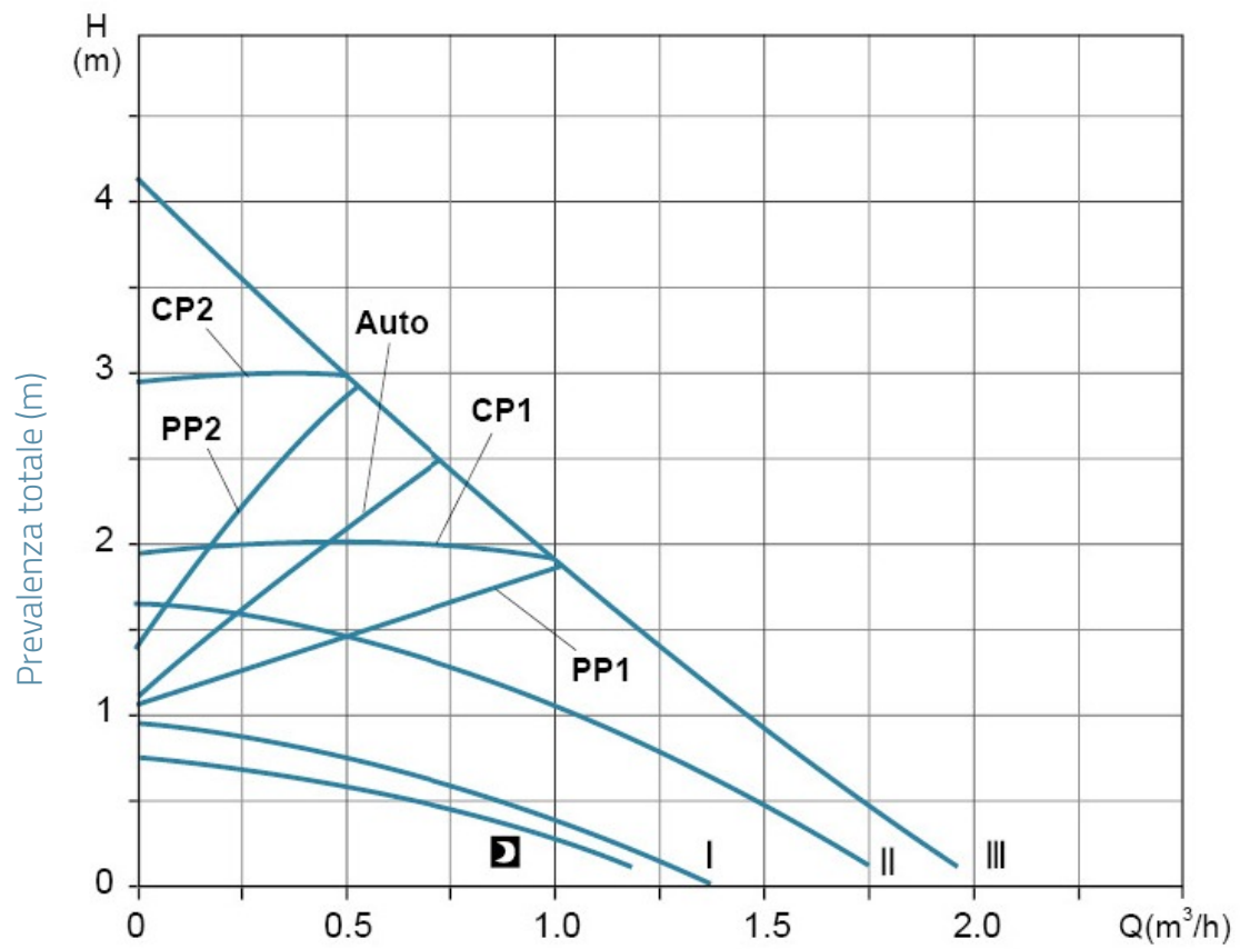
ARPXX-40 Q-H
